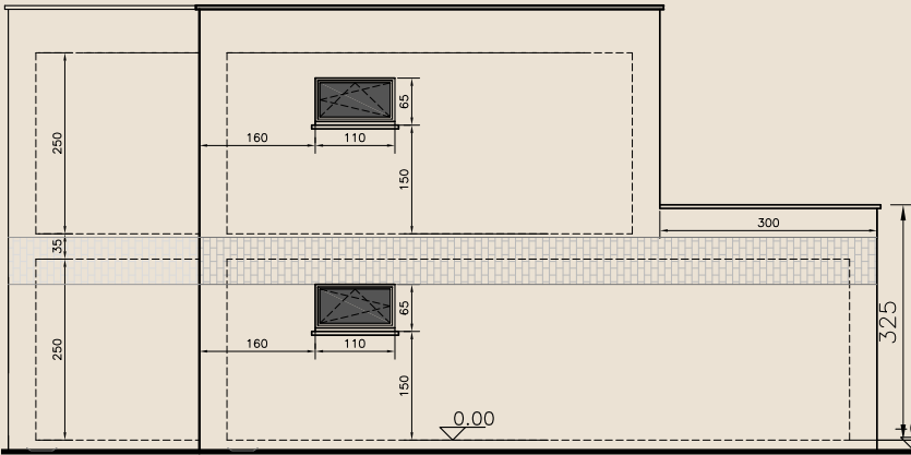
Zijgevel rechts
