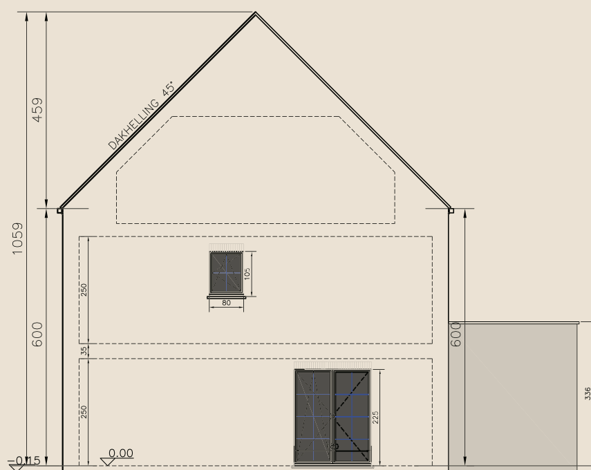
Zijgevel
