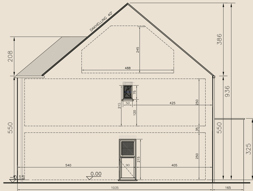
Zijgevel rechts
