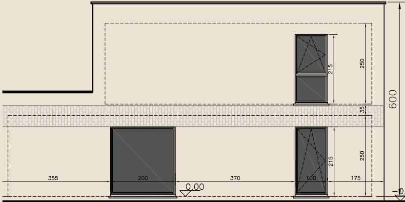
Zijgevel links
