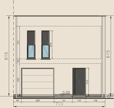
Voorgevel
