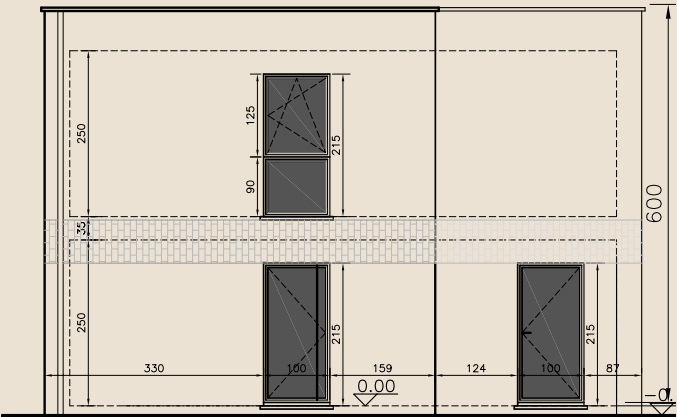
Achtergevel
