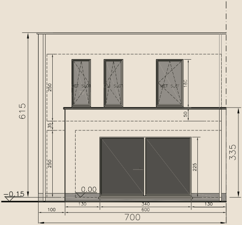
Achtergevel
