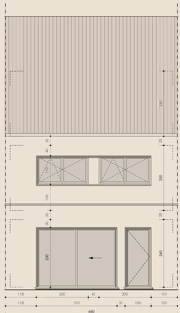
Achtergevel
