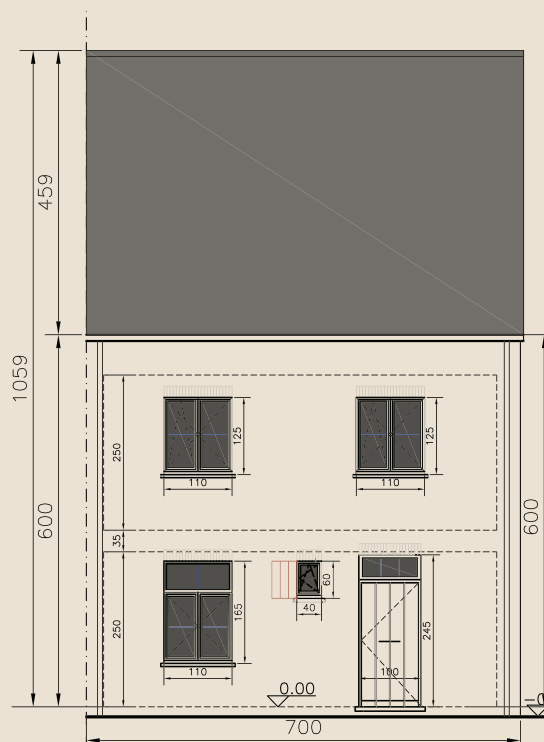
Voorgevel
