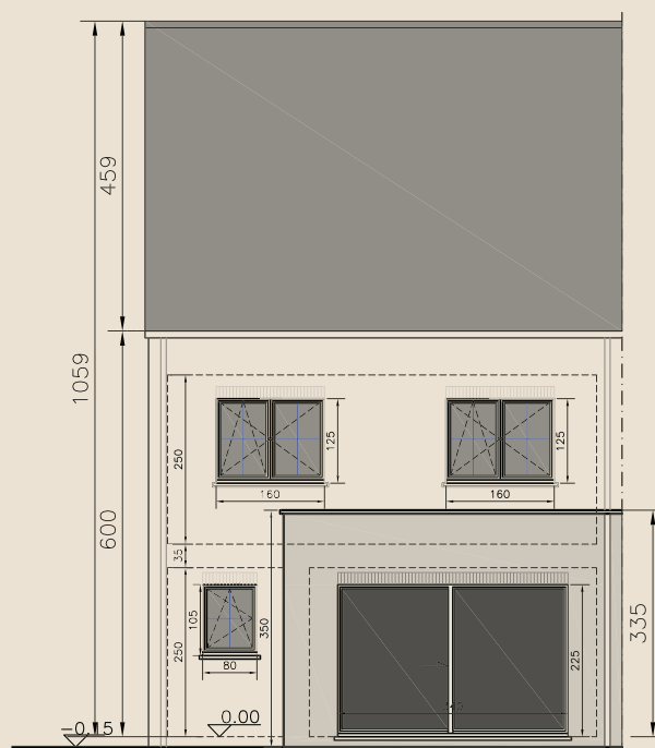
Achtergevel
