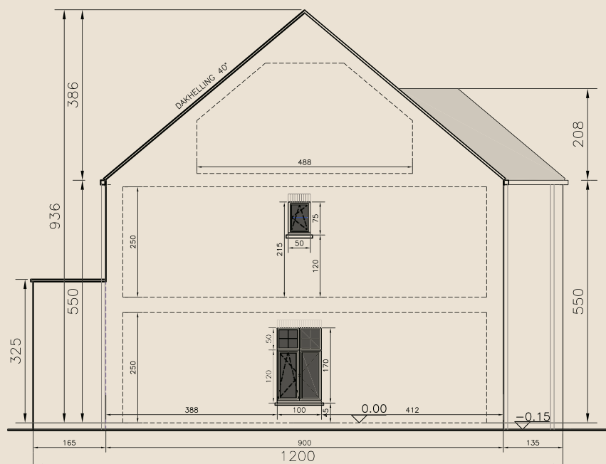
Zijgevel links
