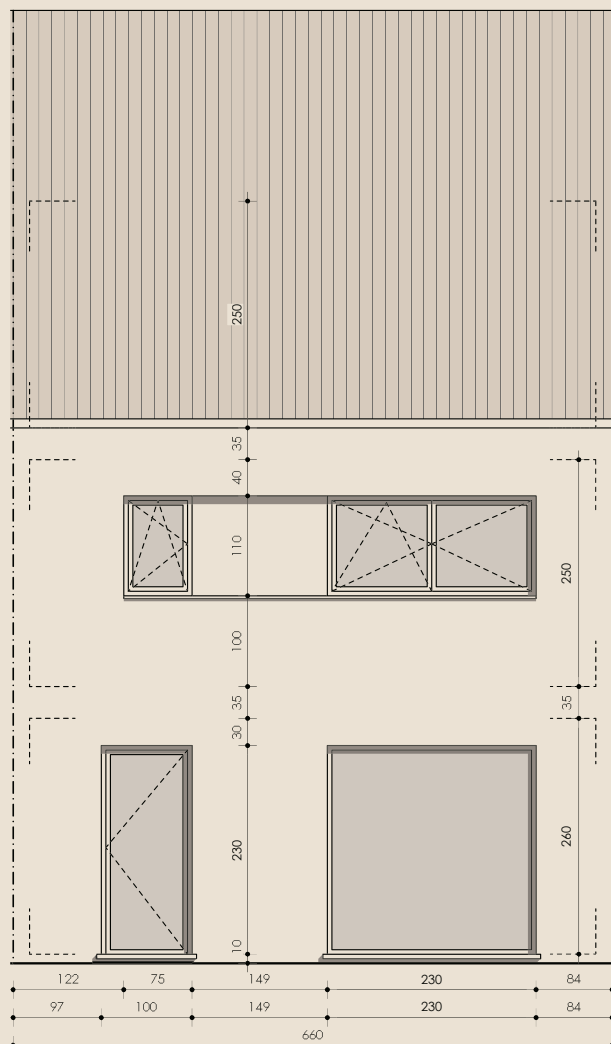
Voorgevel
