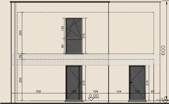
Voorgevel
