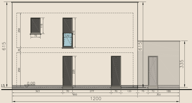
Zijgevel
