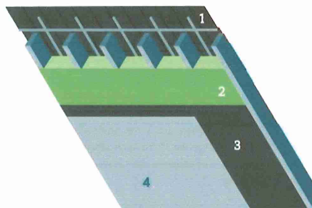
1. Onderdak | 2. Isolatie | 3. Dampscherm | 4. binnenaftrekking
