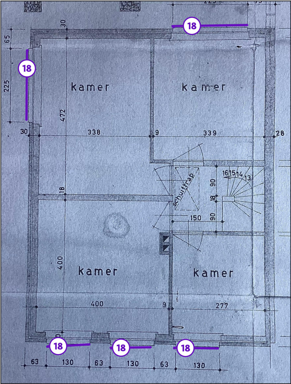
Legende van plan 1.6: Eerste verdiep
